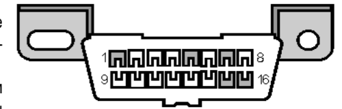
рис.11 Контакты колодки OBD II
