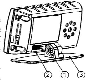
рис.5 Крепление БК на панель приборов
